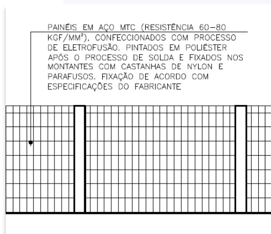
Figura 8 - Exemplo de Detalhamento de Gradil
