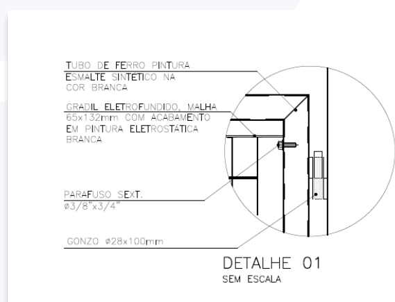
Figura 8 - Exemplo de Detalhamento de Gradil
